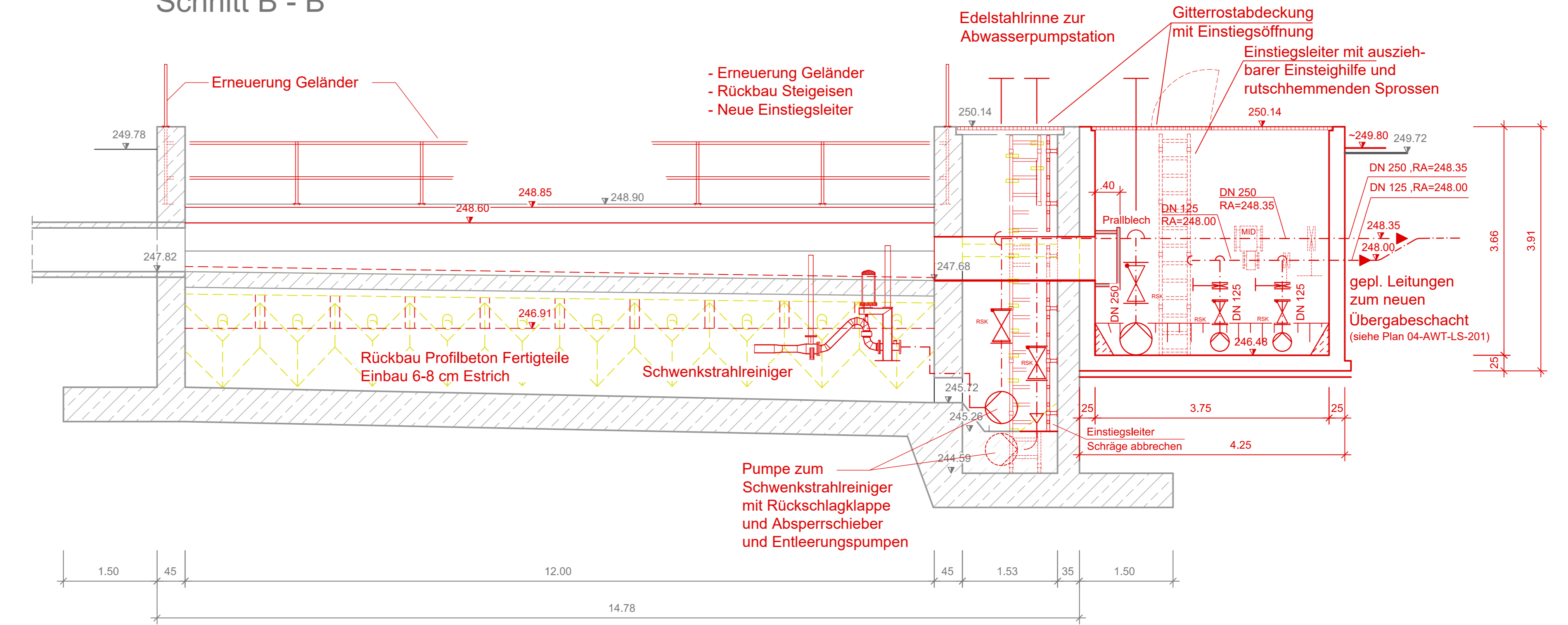
Schnitt B - B
