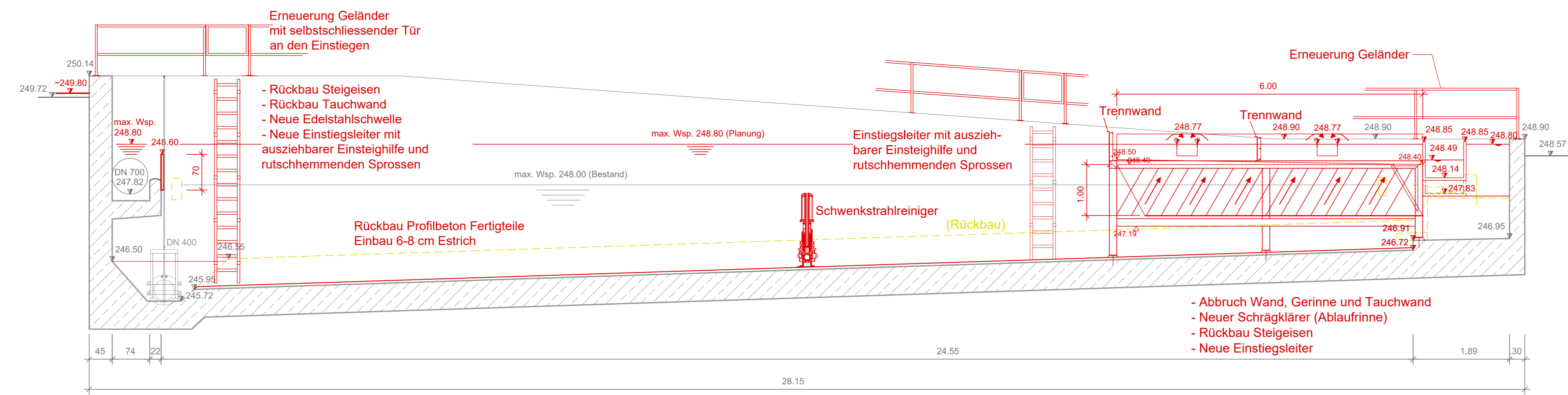
Schnitt A - A
